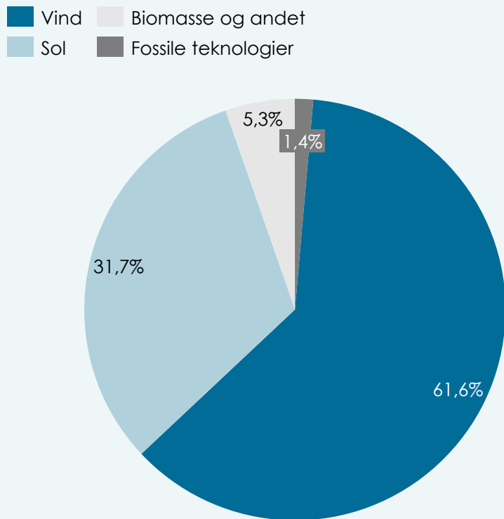
Andel af samlet produktion på tværs af produktionsteknologier i 'Business as usual' % af samlet elproduktion, 2035
