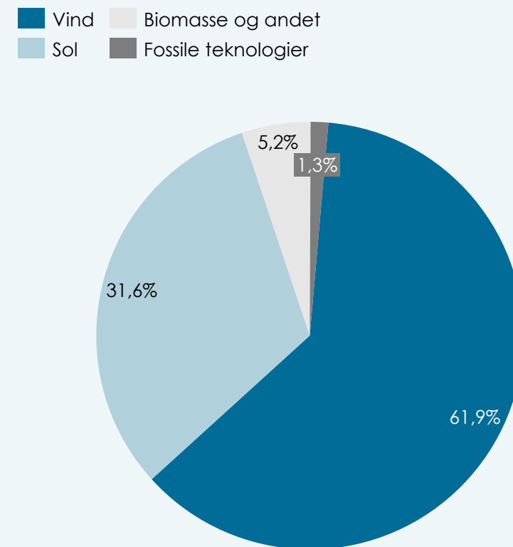
Andel af samlet produktion på tværs af produktionsteknologier i 'Fuldt fleksibelt forbrug' % af samlet elproduktion, 2035
